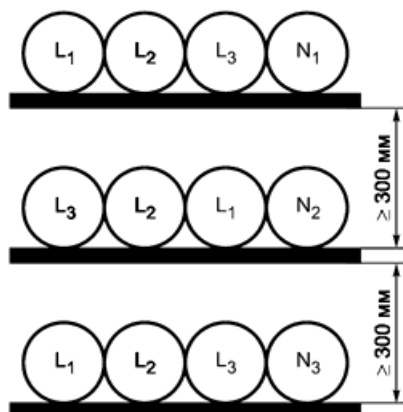
Рисунок Н.52.4 - Специальная конфигурация для девяти параллельных одножильных кабелей в горизонтальной плоскости (см. 523.7)
