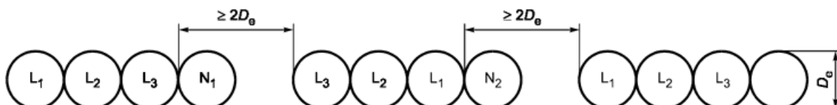
Рисунок Н.52.3 - Специальная конфигурация для шести параллельных одножильных кабелей, уложенных треугольником (см. 523.7)
