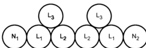
Рисунок Н.52.2 - Специальная конфигурация для шести параллельных одножильных кабелей один выше другого (см. 523.7)
