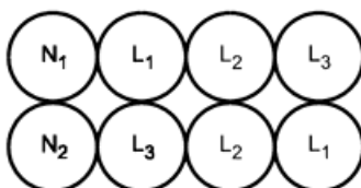
Рисунок Н.52.1 - Специальная конфигурация для шести параллельных одножильных кабелей в горизонтальной плоскости (см. 523.7)
