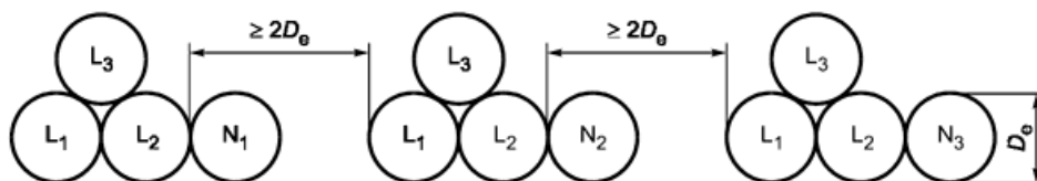
Рисунок Н.52.5 - Специальная конфигурация для девяти параллельных одножильных кабелей один выше другого (см. 523.7)
